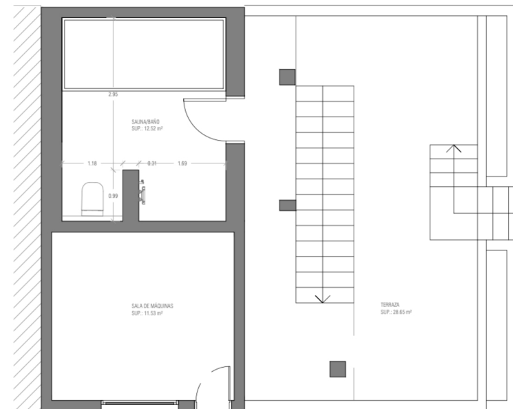
PLANTA SEMISÓTANO
