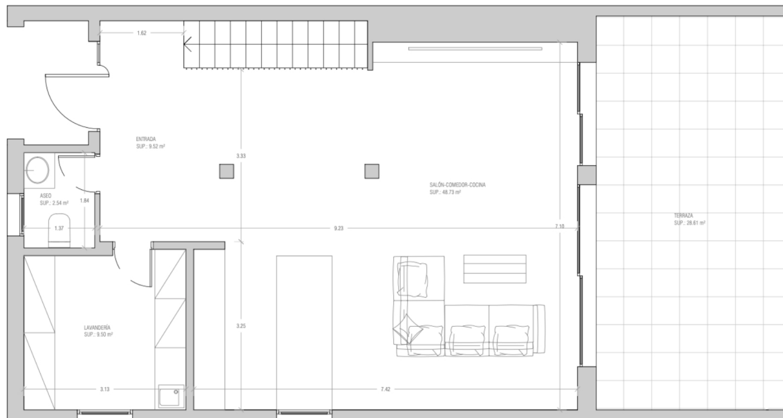
PLANTA PISO
