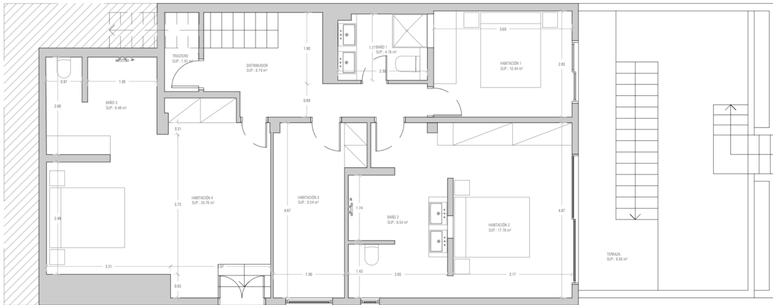
PLANTA BAJA
